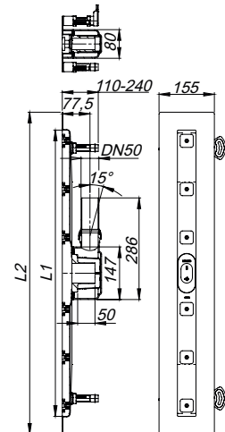
douchegoot CeraLine F 500 – 1200
